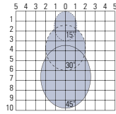
7 meter montagehoogte Instelhoek 15°–45°
