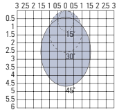
2,5 meter montagehoogte Instelhoek 15°–45°
