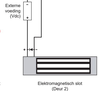
Sluitplaat (Deur 1)
