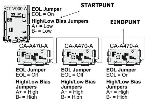
Figuur 2: Jumpers instellen
