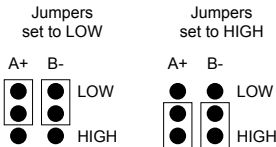
Figuur 3: Jumpers A+ en B- instellen
